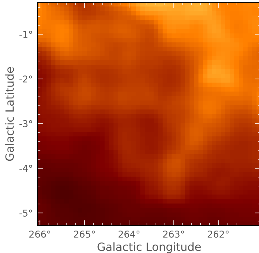
Fermi Tools Background
